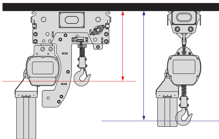
低举型链条葫芦
