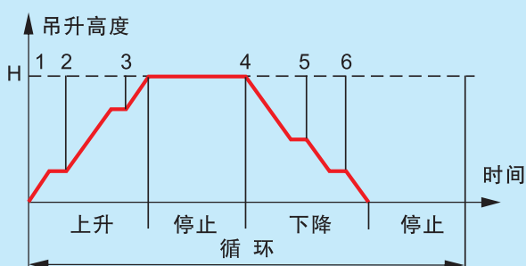
吊升单速
