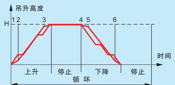
吊升双速
